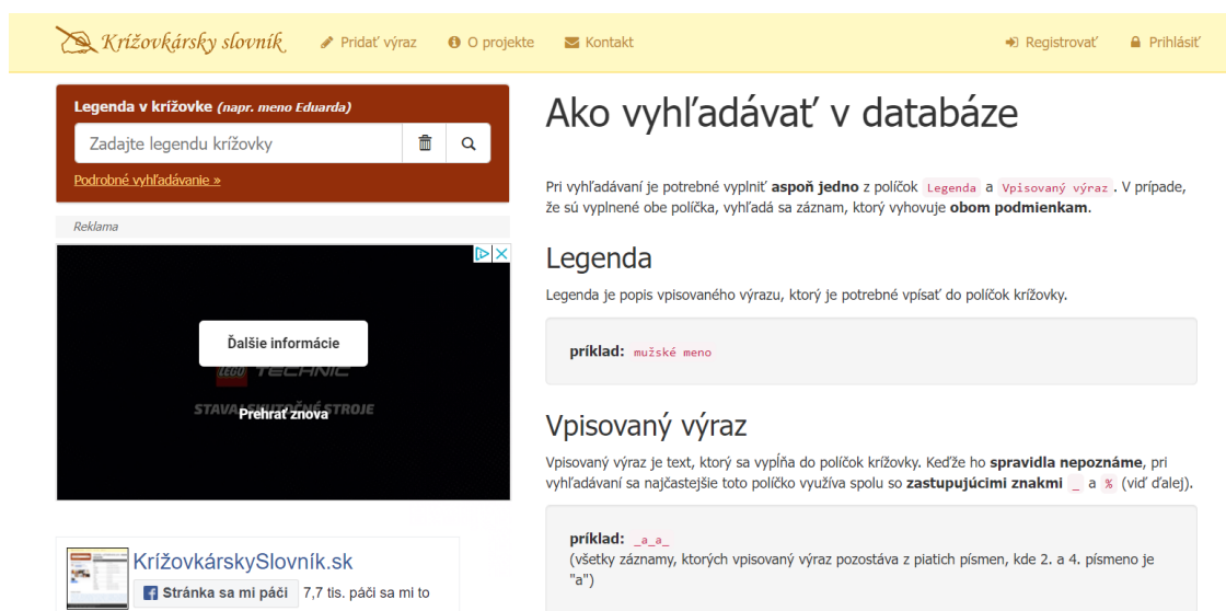
Obrázok 98 - Krížovkársky slovník
