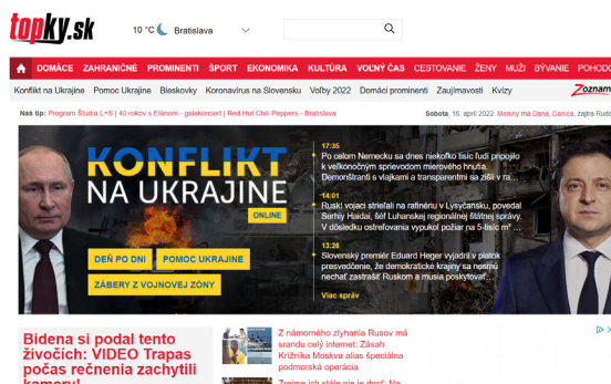
Obrázok 67 – www.topky.sk
