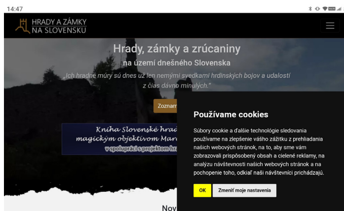
Obrázok 25 – Cookies
