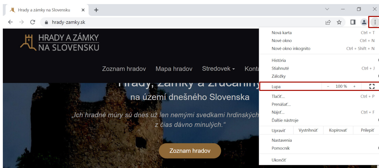
Obrázok 31 – Lupa – 100 %
