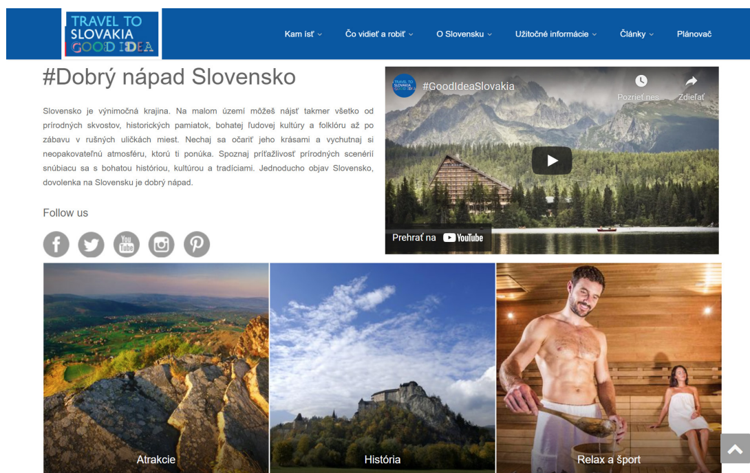
Obrázok 91 – slovakia.travel
