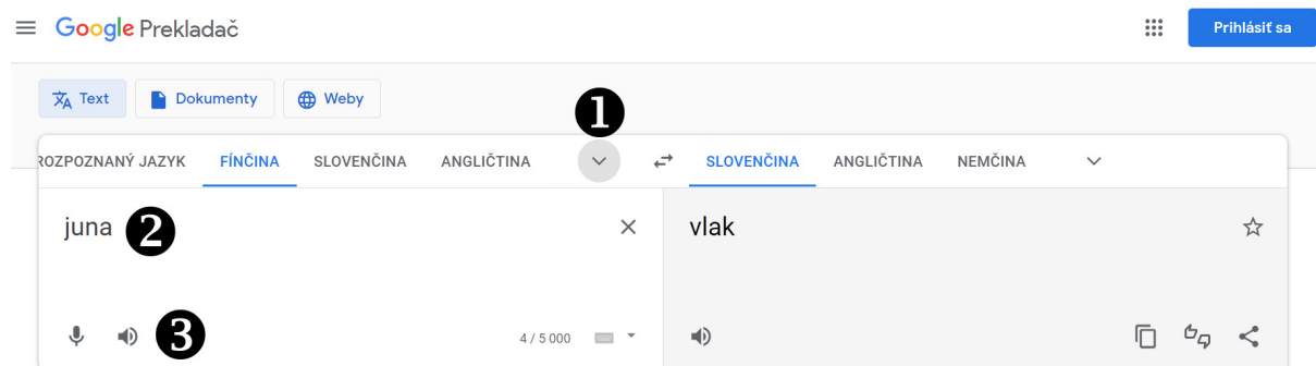
Obrázok 102 - Prekladač
