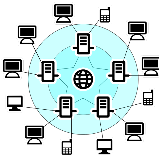
Obrázok 1 – Internet
