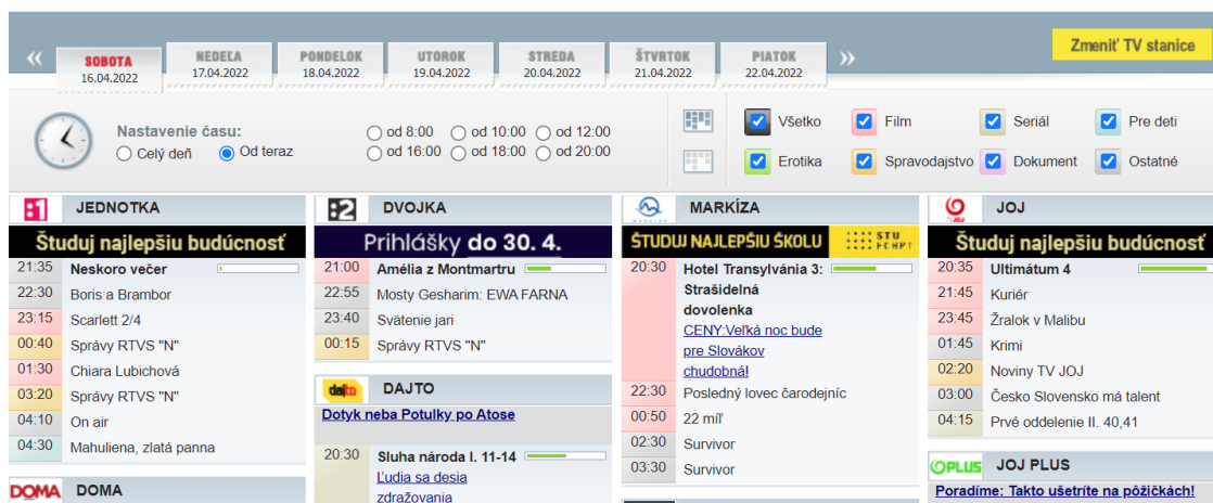
Obrázok 72 – tv-program.sk
