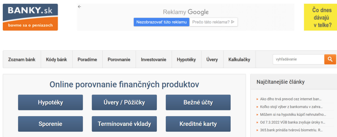
Obrázok 76 – www.banky.sk
