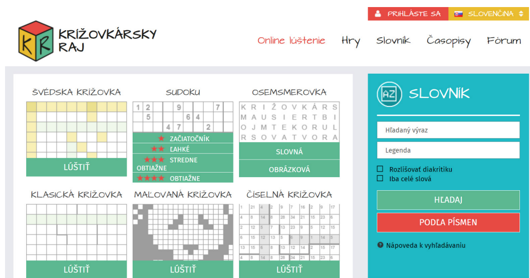
Obrázok 97 – Krížovkársky raj
