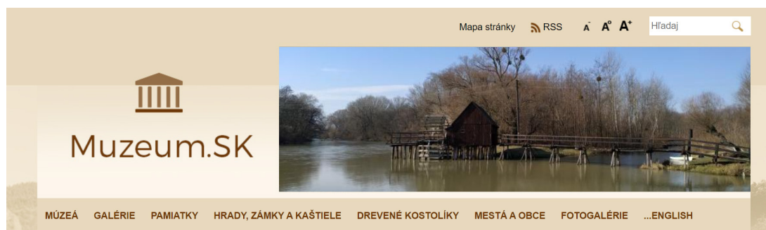
Obrázok 90 – www.muzeum.sk
