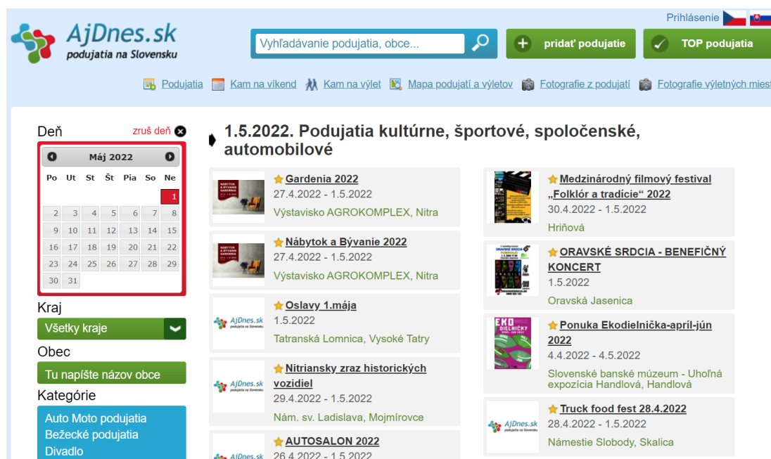
Obrázok 87 – www.ajdnes.sk
