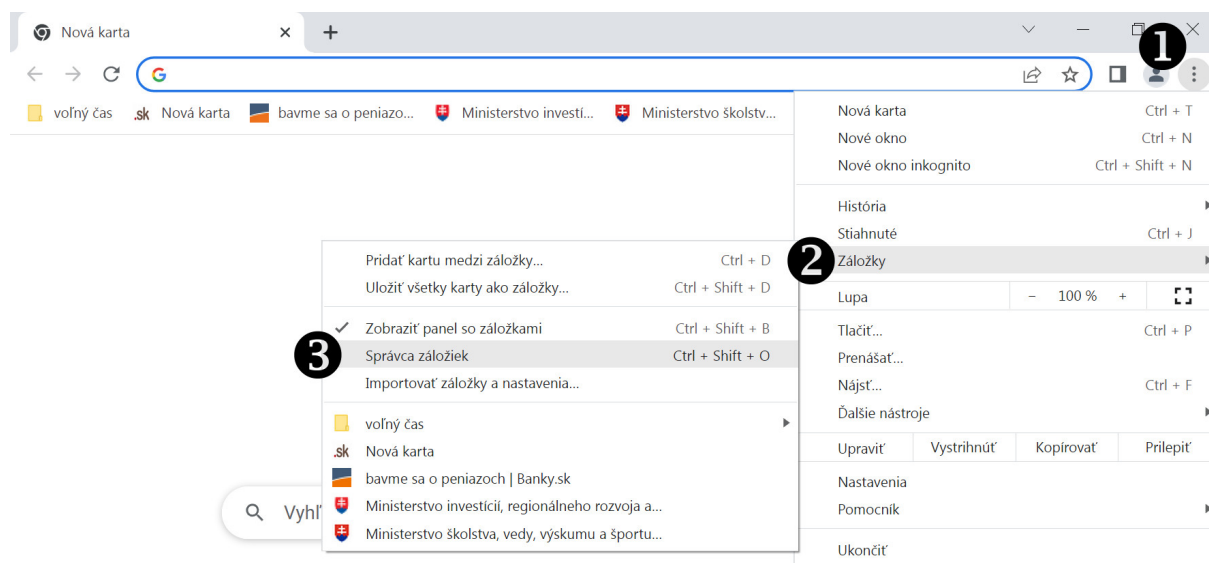
Obrázok 44 – Správca záložiek
