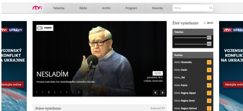
Obrázok 71 – Stránka www.rtvs.sk
