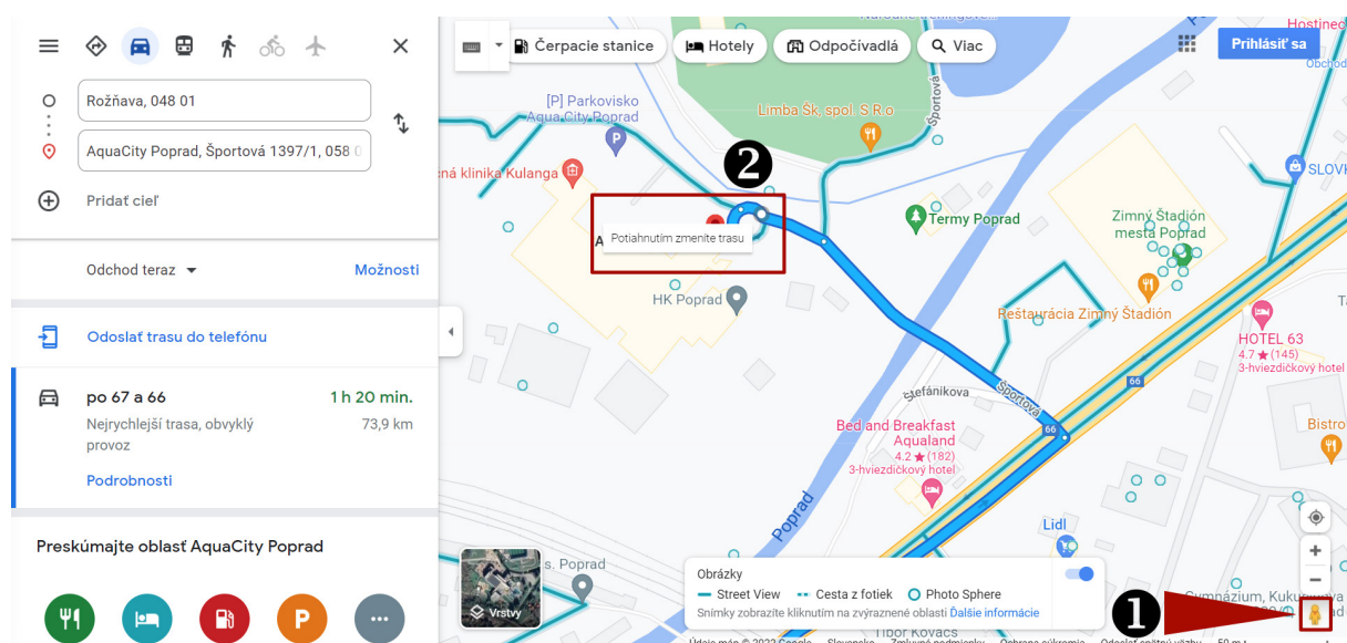
Obrázok 93 – Zapnutie streetview
