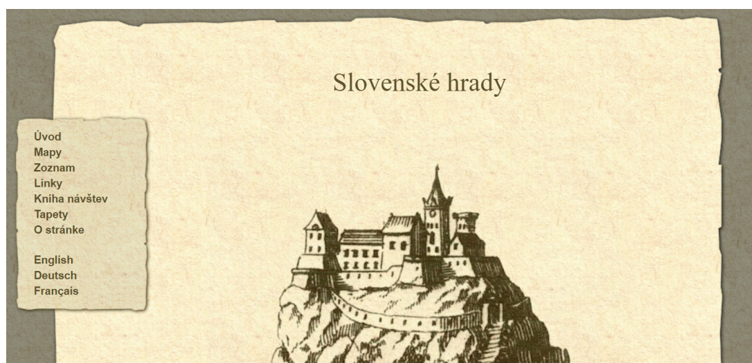
Obrázok 89 – slovenskehrady.sk
