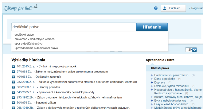
Obrázok 85 – www.zakonypreludi.sk
