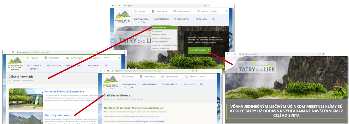
Obrázok 6 – Hypertextové odkazy
