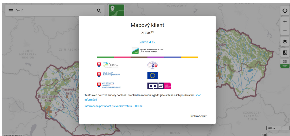
Obrázok 78 – zbgis.skgeodesy.sk
