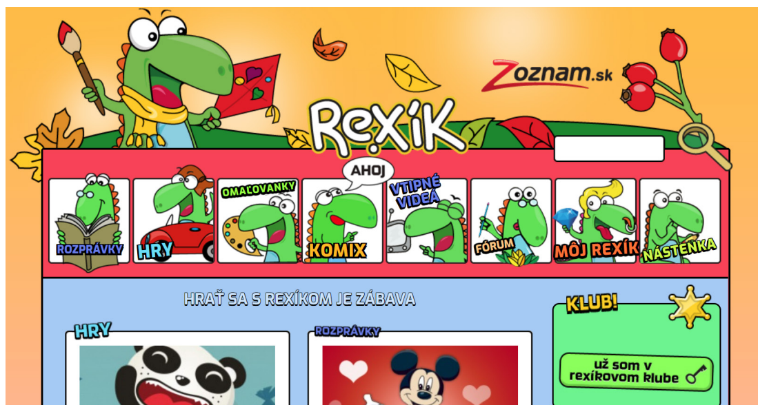
Obrázok 99 - rexik.sk
