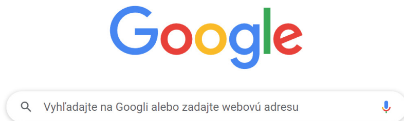
Obrázok 49 – Vyhľadávač Google
