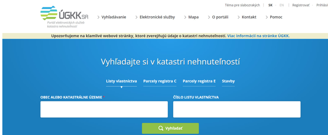
Obrázok 77 – kataster.skgeodesy.sk
