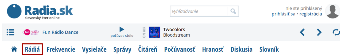
Obrázok 68 – www.radia.sk
